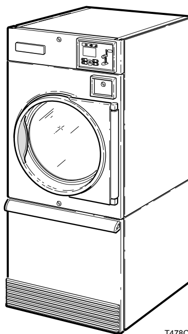
T478C
